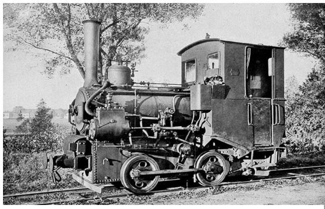
Lokomotywa nr 43 "kolejki buraczanej", Cukrowni Klecina 1920r. (źródło: www.dolnyslask.org.pl)
